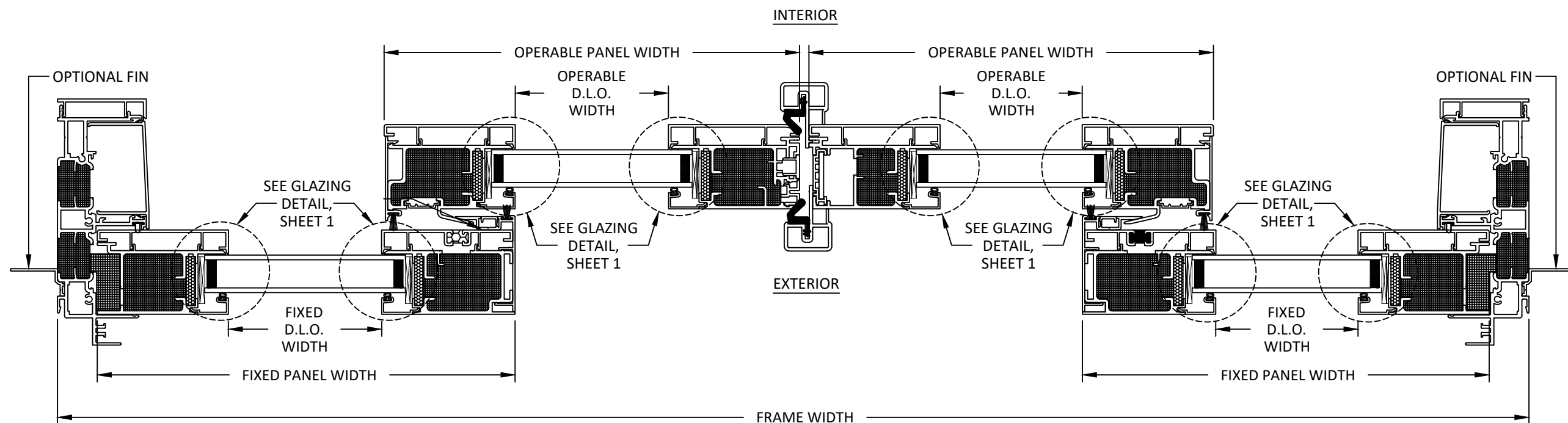
B HORIZONTAL SECTION 6 OXXO
