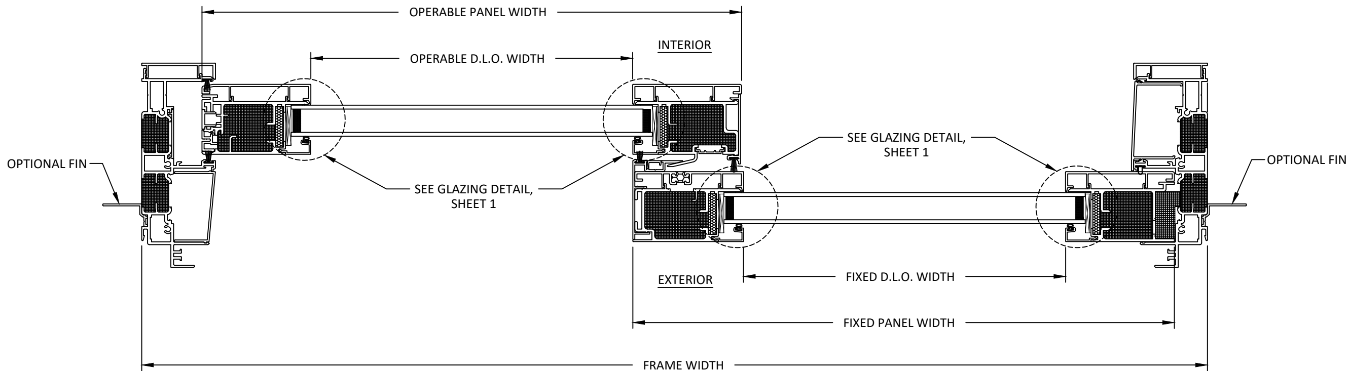
A HORIZONTAL SECTION 6 XO
