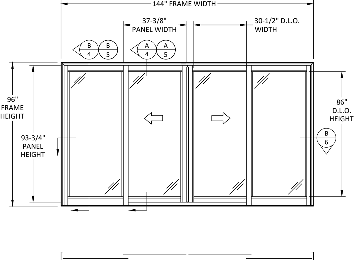
ELEVATION
